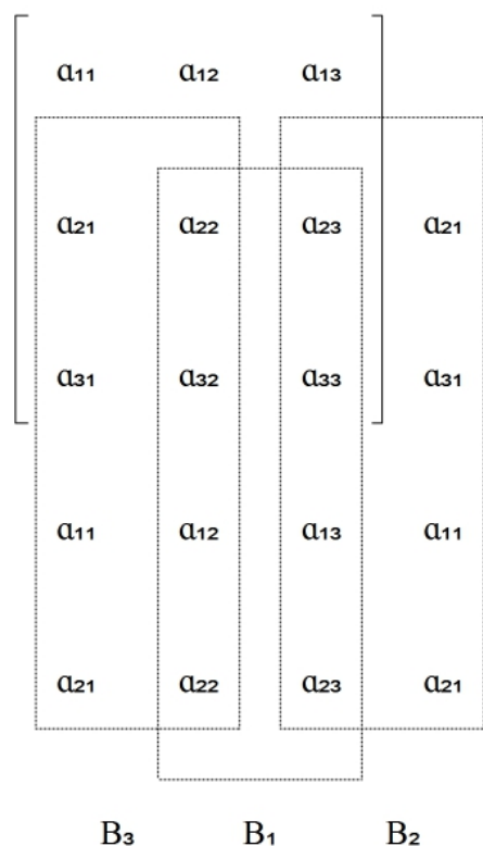
Figura 1: Matriz \mathbf{A} y bloques auxiliares \mathbf{B}_1, \mathbf{B}_2, \mathbf{B}_3
